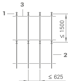
Module 1250 x 625 mm
