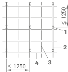
Module 600 x 600 mm
