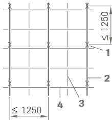
Module 625 x 625 mm
